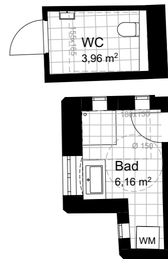
VARIANTE BARRIEREFREIE SANITÄRRÄUME M 1:100
