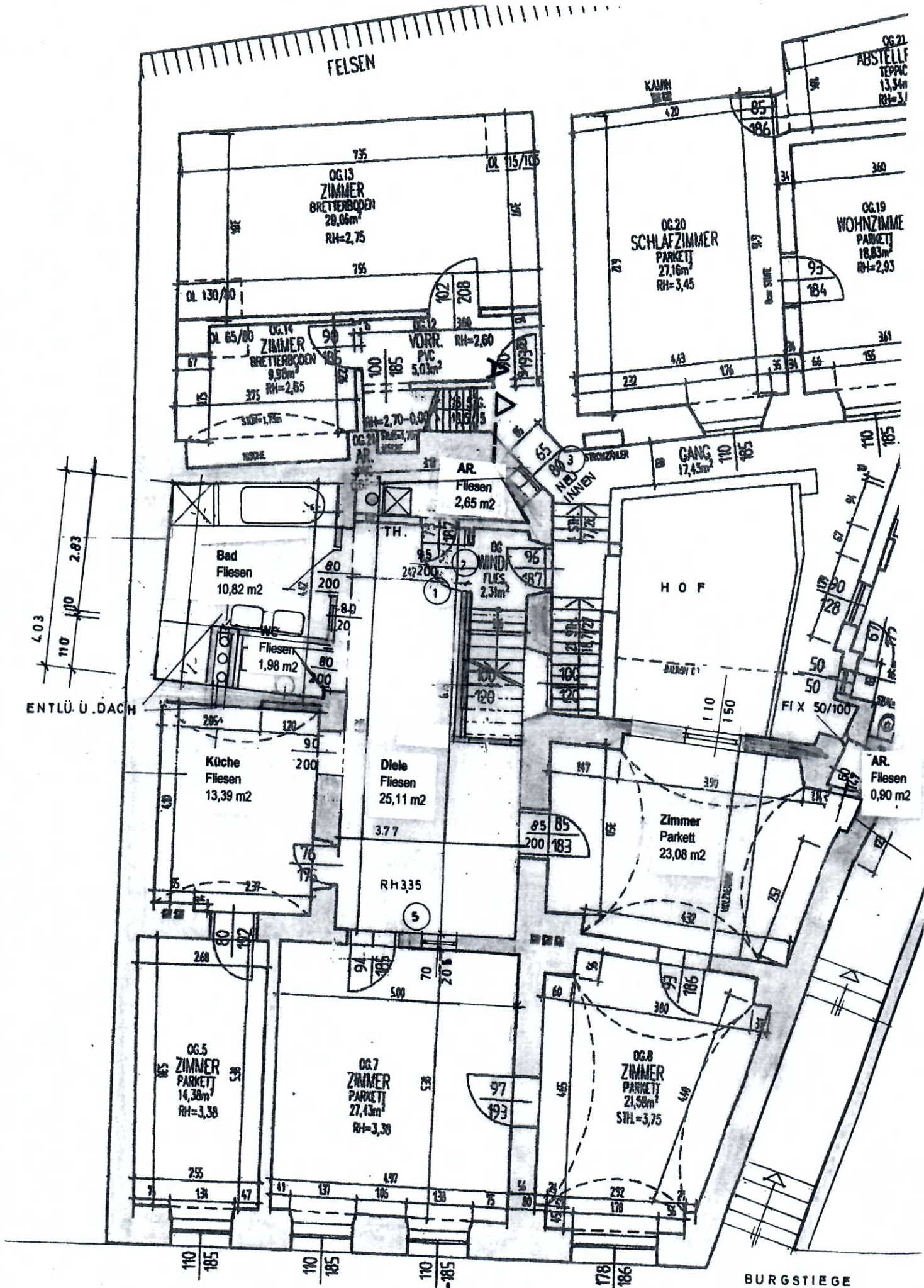
1. OBERGESCHOSS M = 1 : 100
