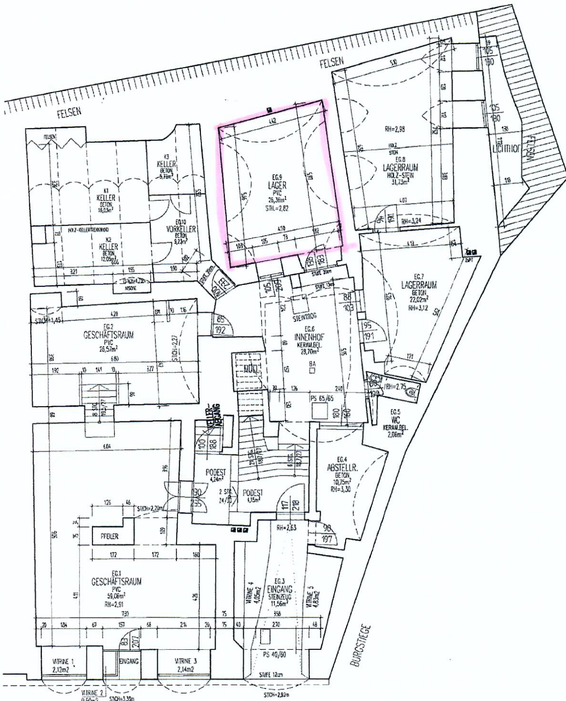
GRUNDRISS ERDGESCHOSS
