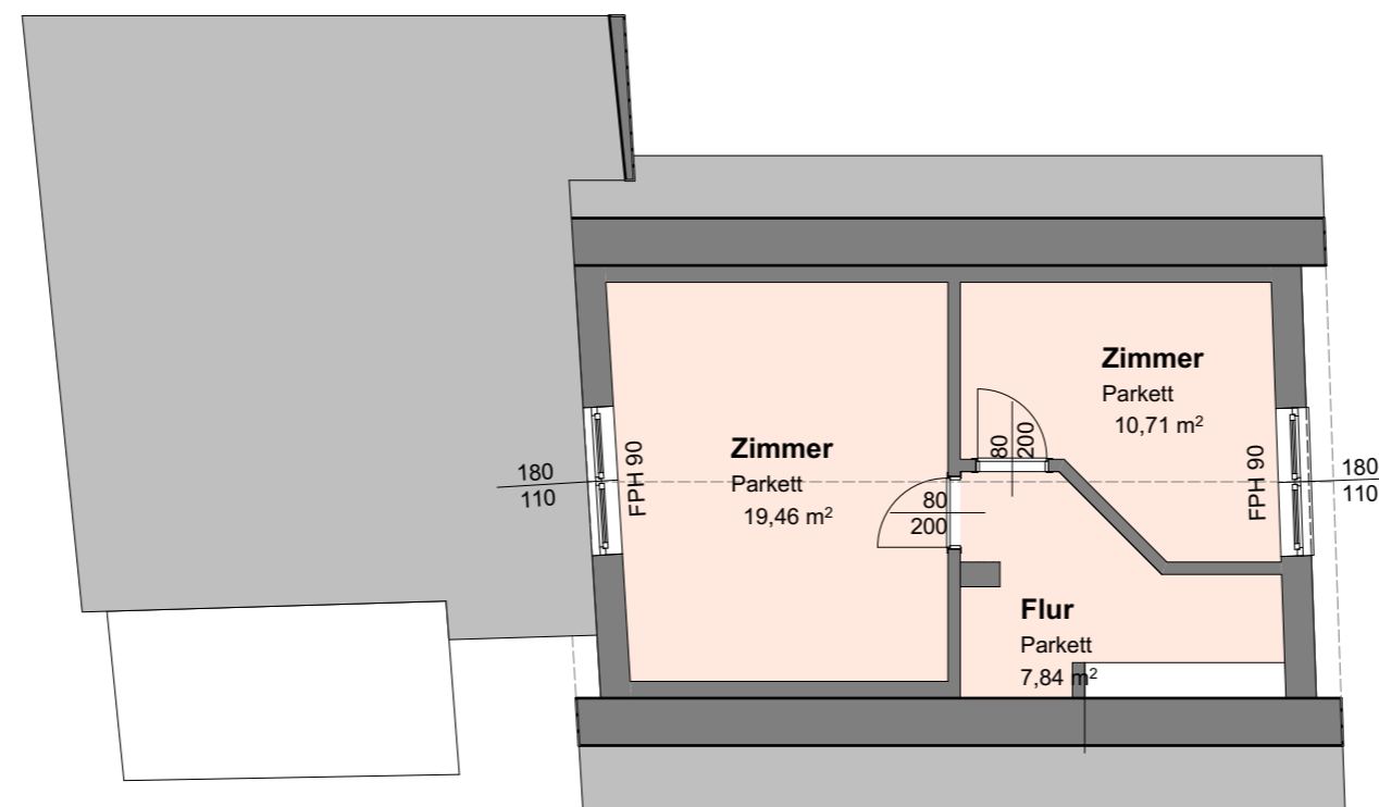
DACHGESCHOSS
