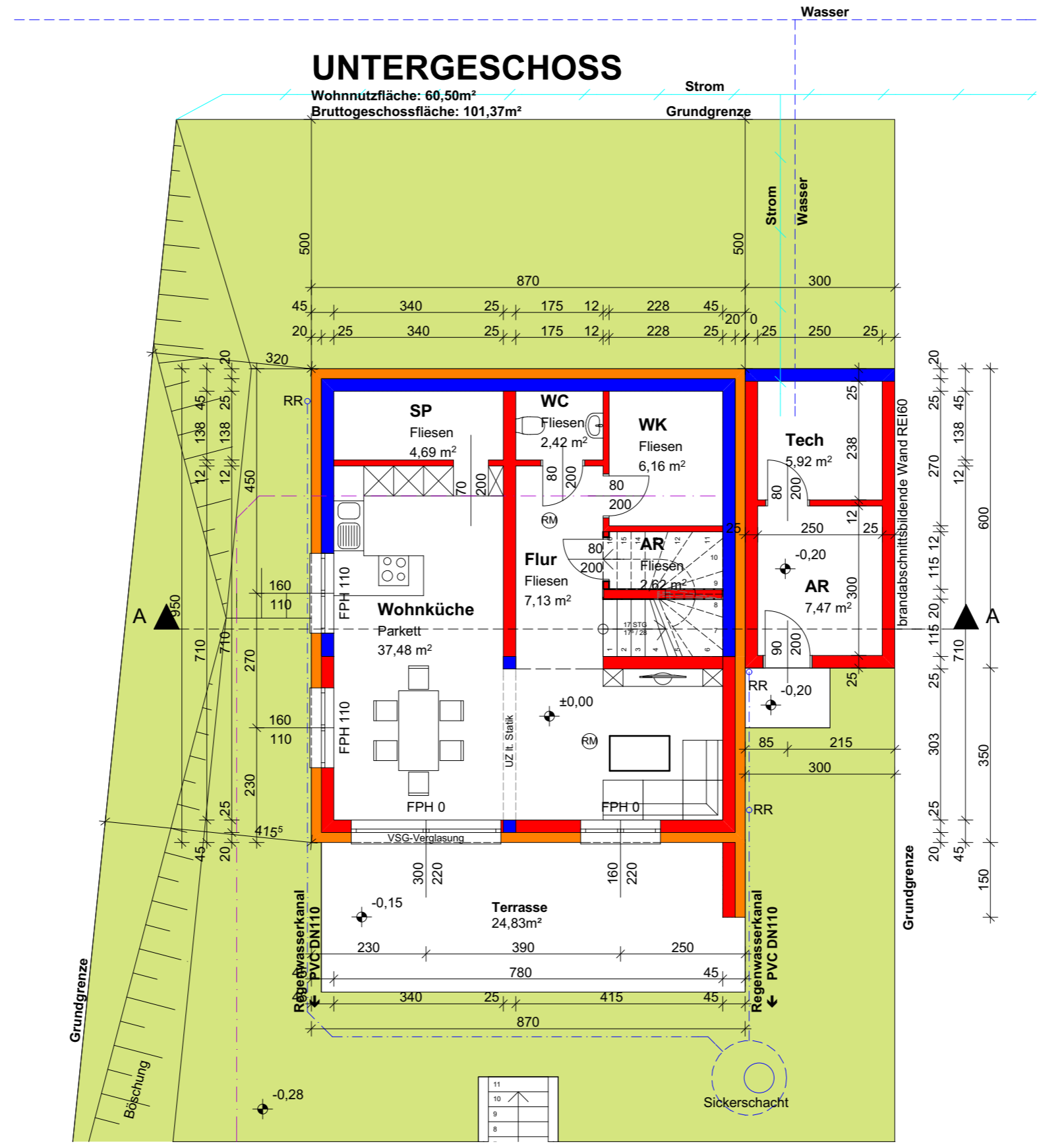
0. Untergeschoss 1:100
